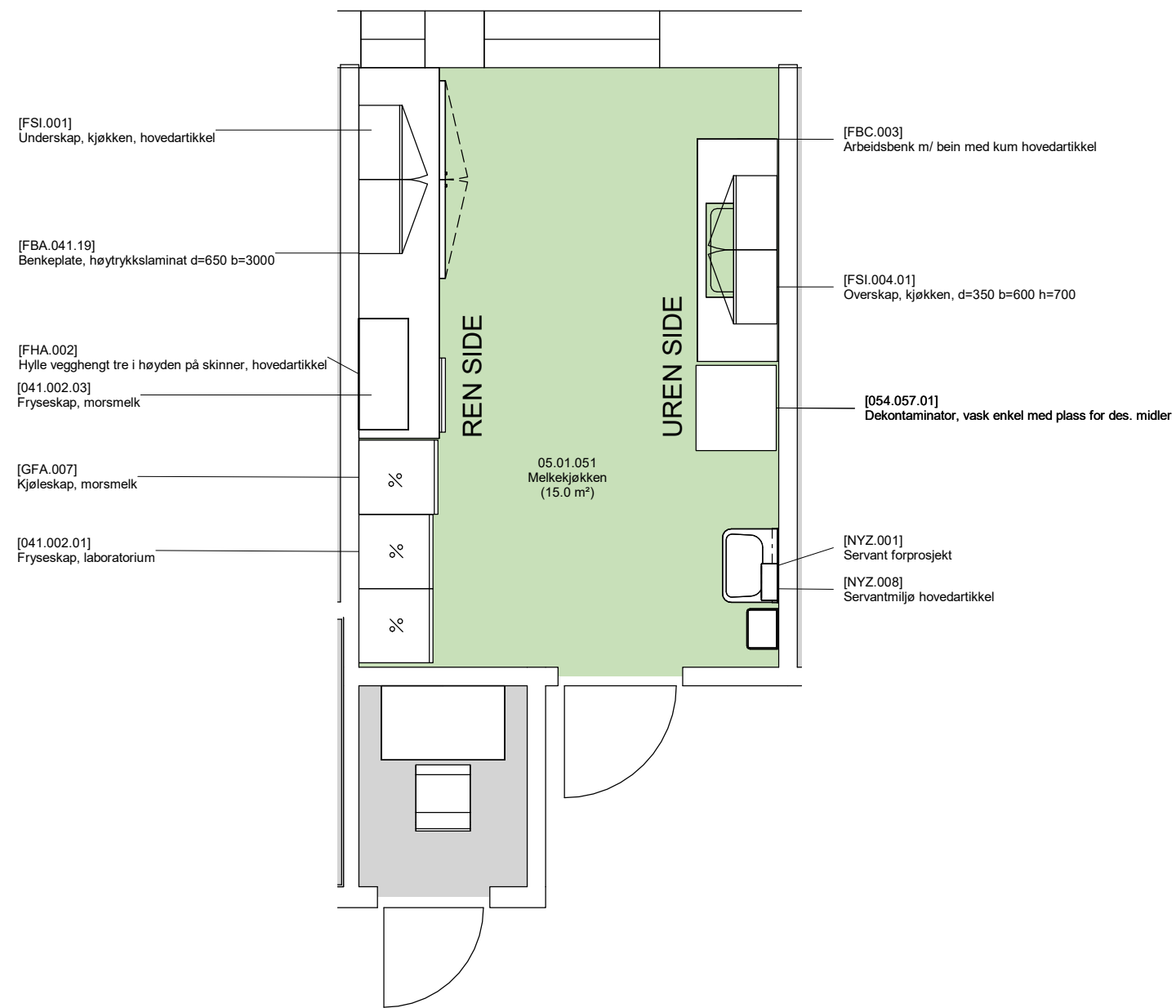
Planutsnitt 05.01.051 Melkekjøkken
