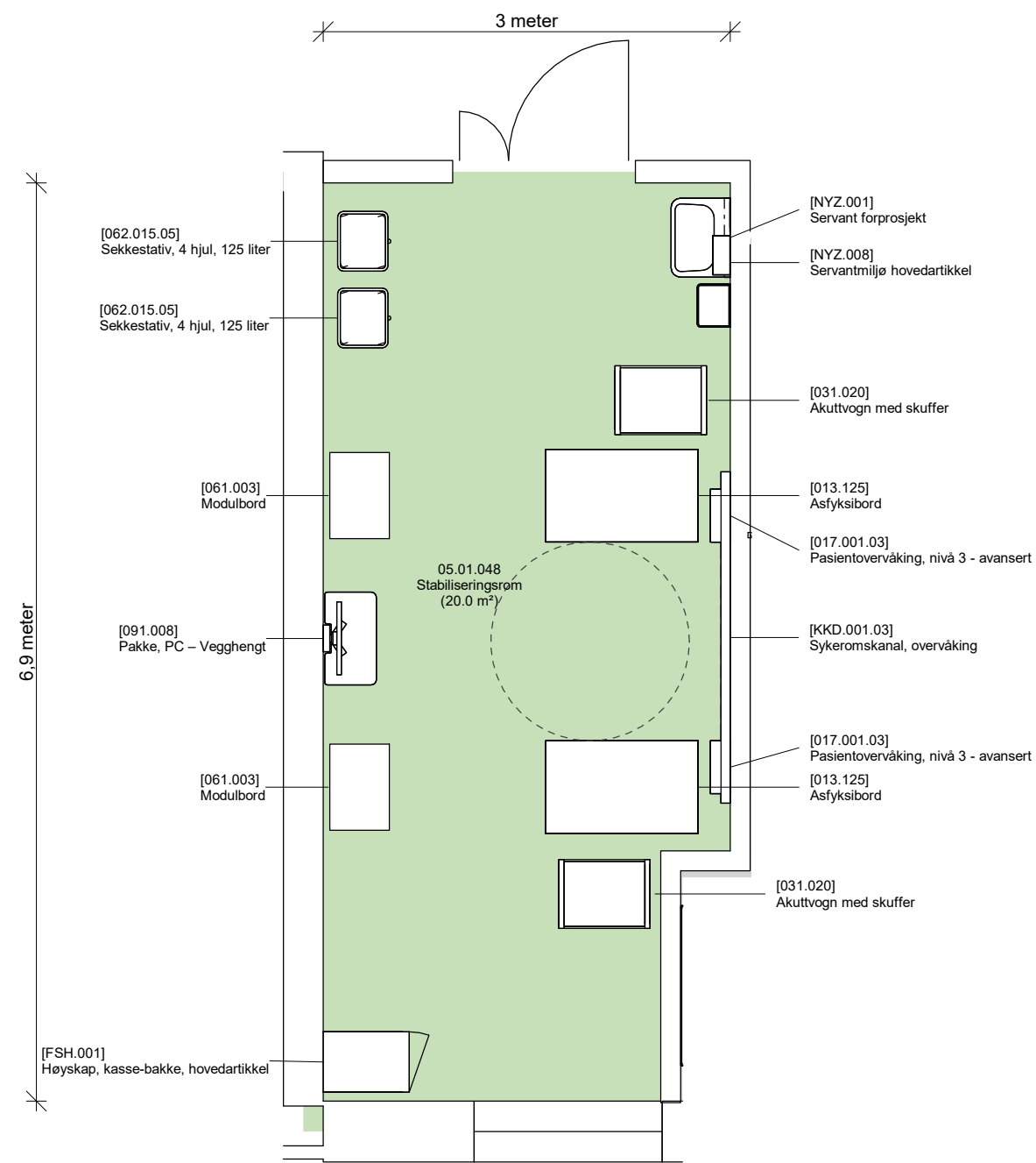
Planutsnitt 05.01.048 Stabiliseringsrom
